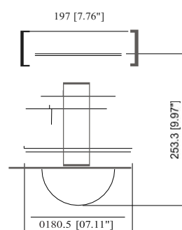
G23(B)-30W~60W
